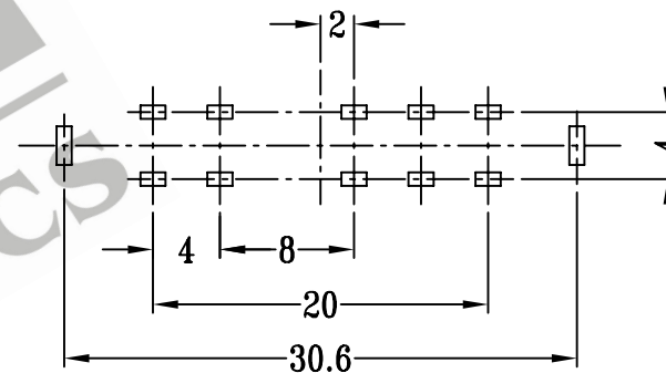
P.C.B LAYOUT
